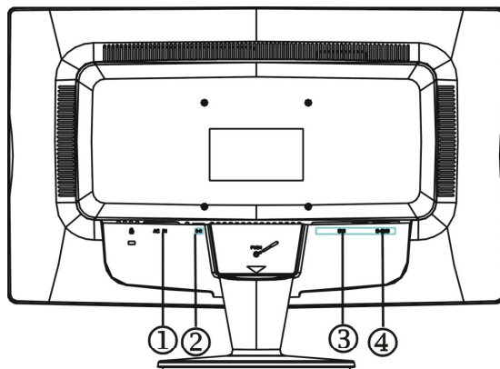
図2 入力端子
